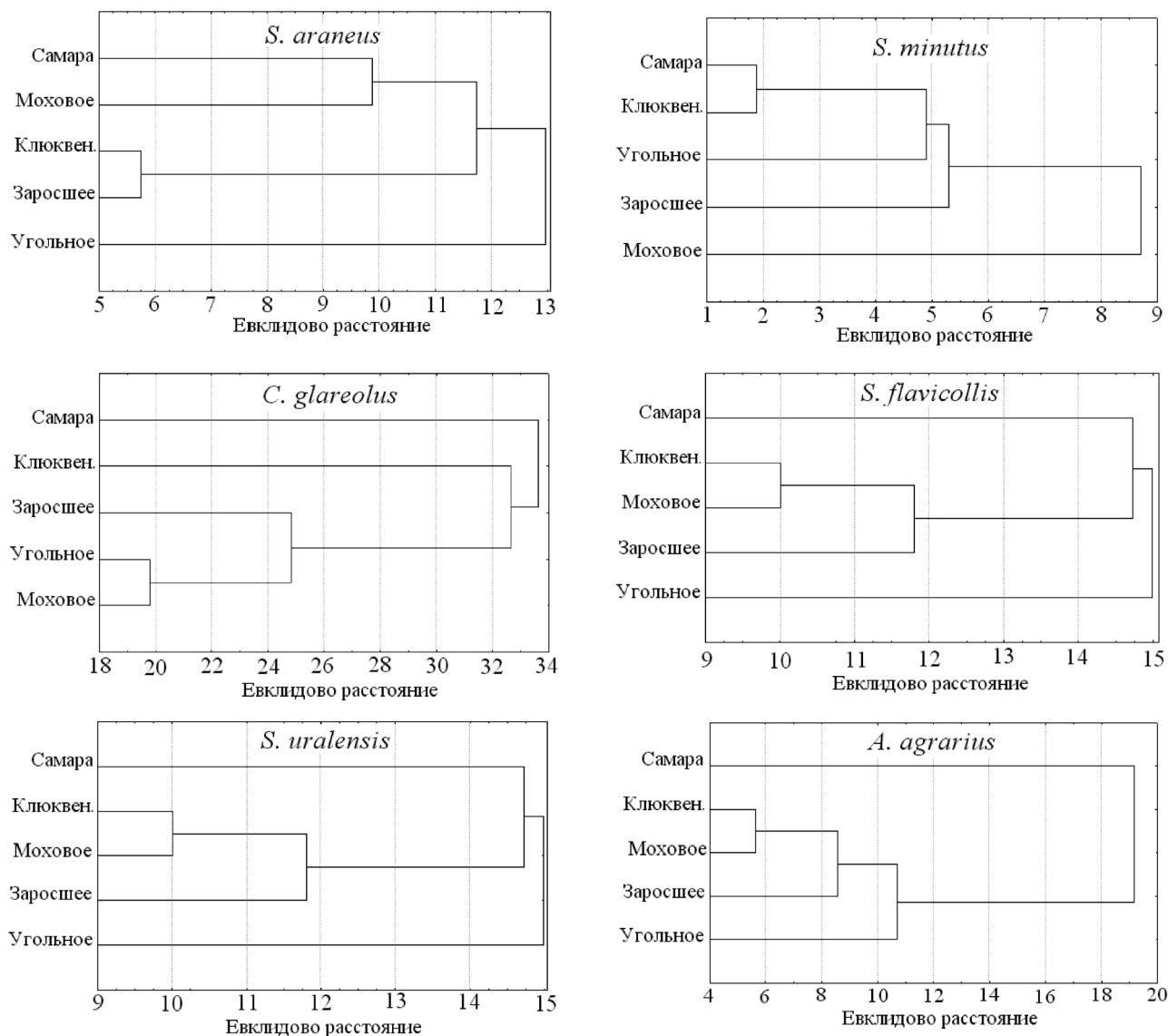
Рис. 2. Взаимосвязи многолетней относительной численности «фоновых» видов мелких млекопитающих Усманского бора в пяти обследованных биотопах окрестностей биоцентра ВГУ «Веневитиново» (1988 – 2011 гг.).
